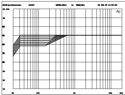
Obr. 6. Vplyv prepínača „bass level“ na frekv. charakteristiku (zjednodušené).
