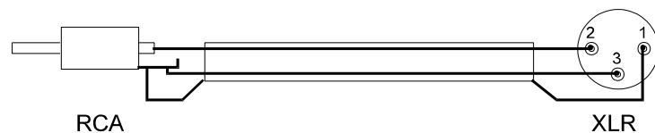
Obr. 2. Kábel pre nesymetrické prepojenie.
