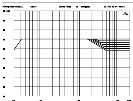
Obr. 4. Vplyv prepínača „treble level“ na frekv. charakteristiku (zjednodušené).
