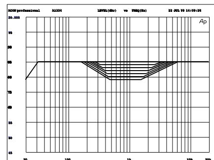
Obr. 5. Vplyv prepínača „mid level“ na frekv. charakteristiku (zjednodušené).
